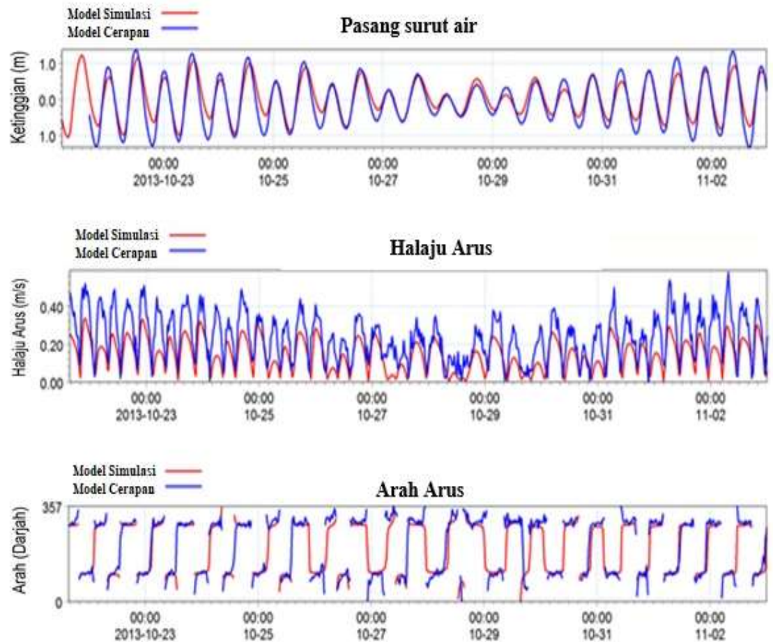
RAJAH 4: Keputusan proses kalibrasi pada pasang surut air, kelajuan dan arah arus
