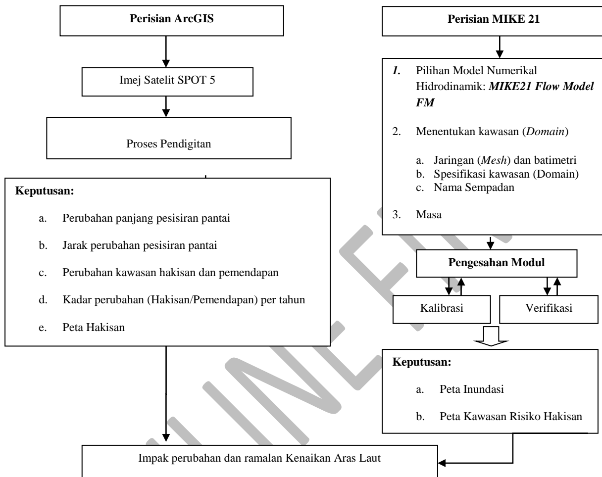
RAJAH 3: Kaedah kajian impak kenaikan aras laut
