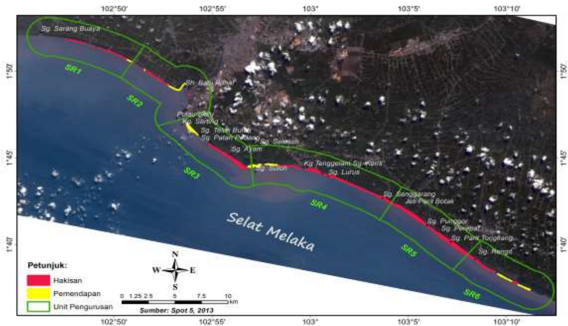
RAJAH 5: Kadar hakisan dan pemendapan
